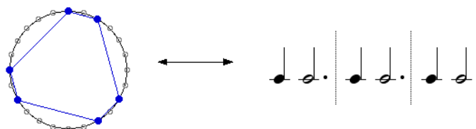
Figure 140 : Mode   transposition limit e correspondant au polyn me Q(x)
