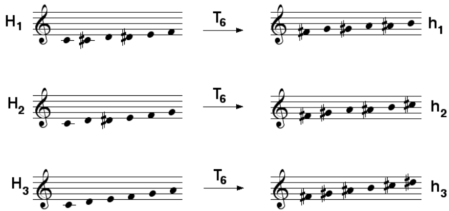
Figure 4 : Les trois hexacordes omni-combinatoires du premier ordre
