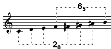
Figure 24 : Le sixième mode représenté avec les deux cribles 2_0 \cup 6_5 ou bien (6_1 \cup 6_3)^c
