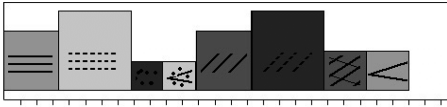
Figure 101 : Complexes sonores associés à l'élément D avec paramètre \alpha
