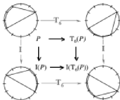
Figure 59 : Un premier réseau transformationnel entre un pentacorde et trois de ses formes
