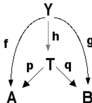
Figure 37 : Diagramme catégoriel pour le produit cartésien
