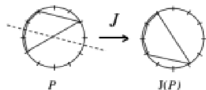
Figure 61 : L'effet de l'opération d'inversion « contextuelle » J
