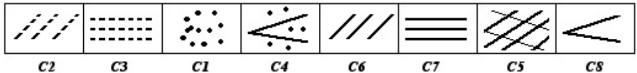
Figure 94 : La séquence initiale des complexes sonores
